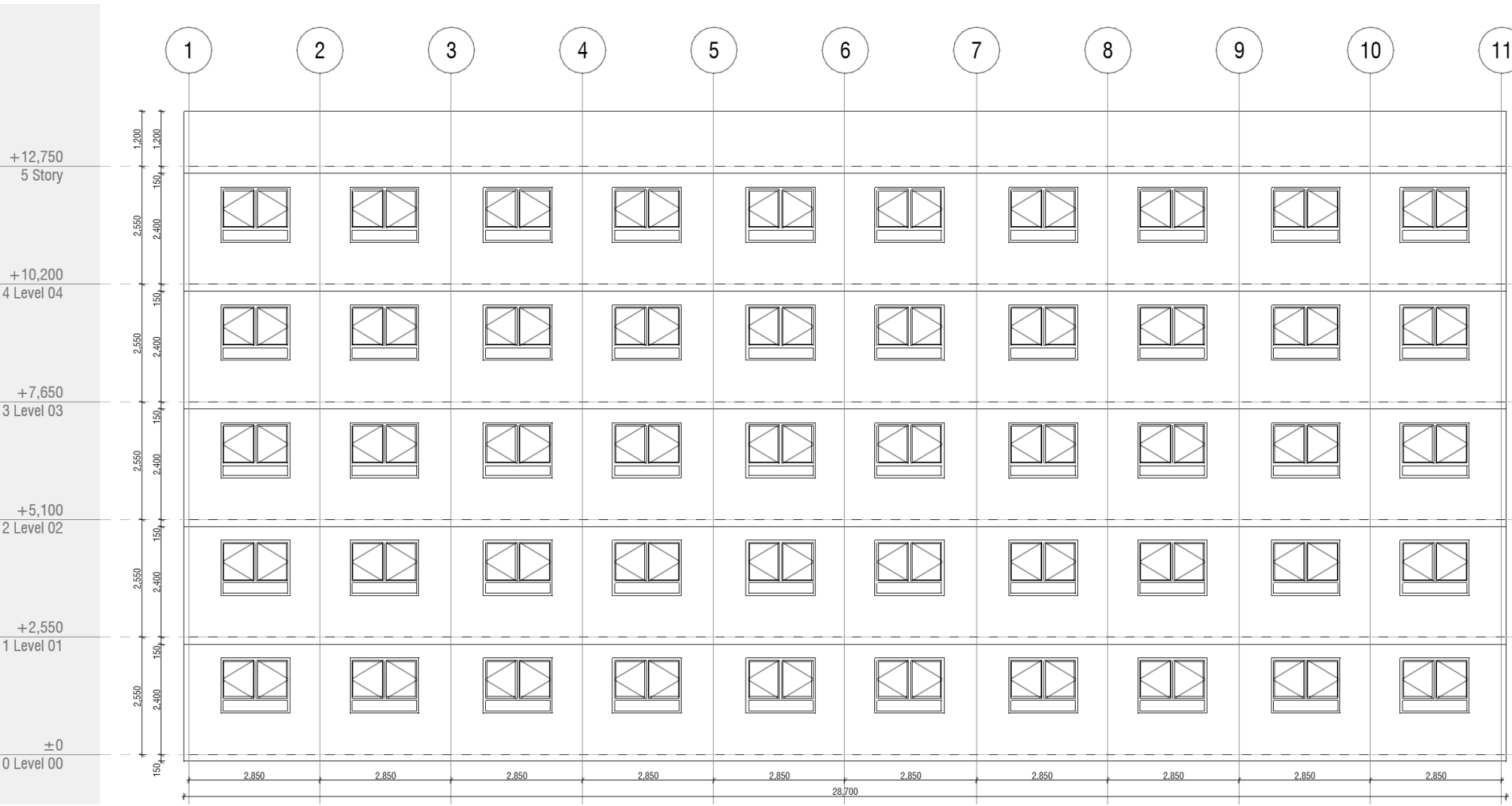
Elevation 01
